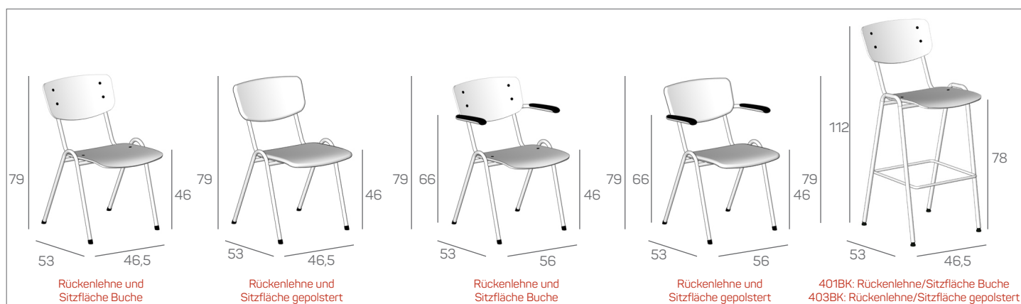
Stuhl 402 lackiert und 404 gepolstert
